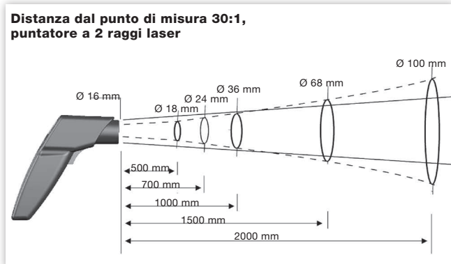
testo 830-T4
